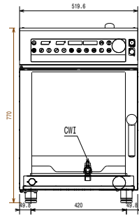
Front aanzicht
