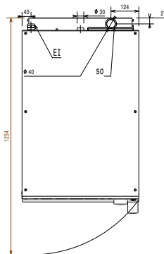
Boven aanzicht
