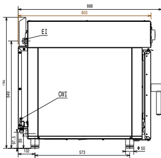
Zij aanzicht
